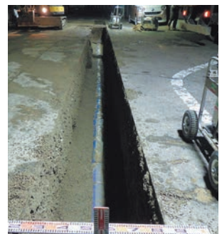
配水管工事
